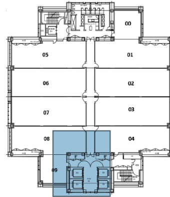
【基準階】
