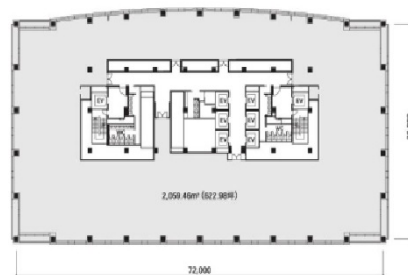
基準階
